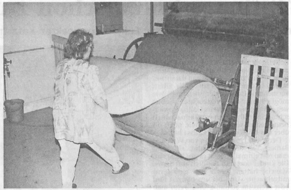
Das Ergebnis des Kardiervorganges ist nach etwa 15 Minuten ein kuschliges Wollvlies, das anschließend weiterverarbeitet wird. Fotos: nic
